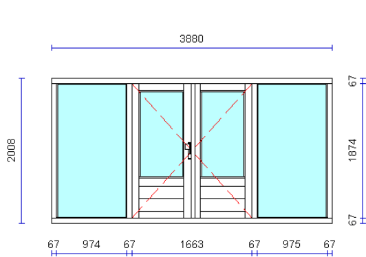
1 1 x Pui openslaande
