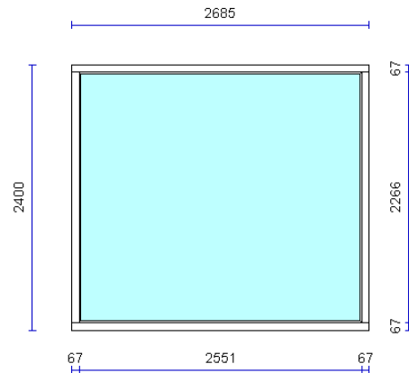
2 1 x Vastkozijn wk
