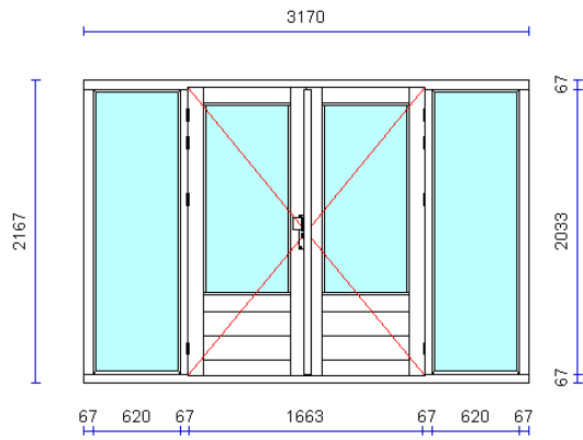
7 1 x Serre openslaande
