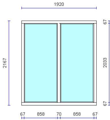
9 1 x Serre pui links vijfver
